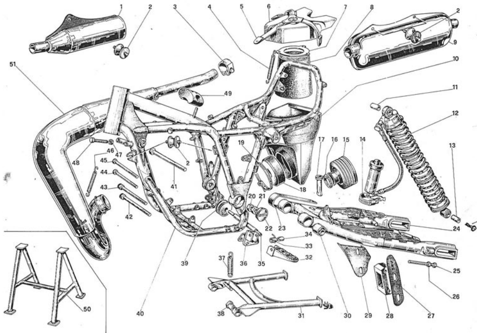
Tav. 5 - Telaio - Cavaletto - Forcellone post. - Ammortizzatori
